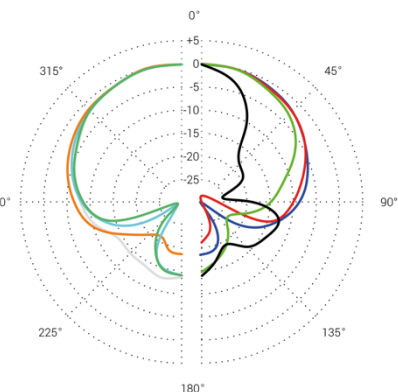
Диаграмма направленности
